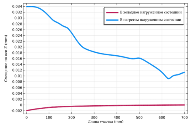
Рисунок 5 – Смещения шпинделя в холодном и нагретом нагруженных состояниях
